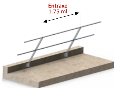
MAK-AN S INCLINÉ 30°
